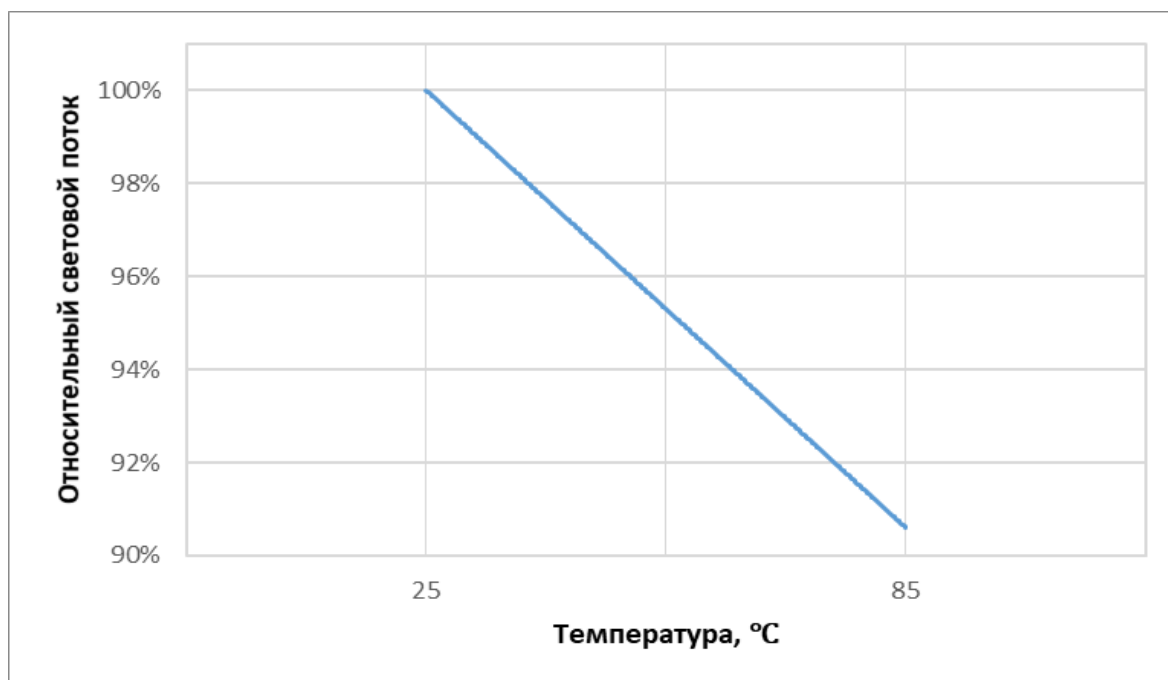
Рисунок 9 – зависимость относительного светового потока от на контактных площадках ( T_s ) при прямом токе = 150 мА ( I_F )
