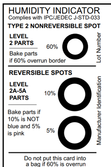
Рисунок 18 – Внешний вид индикатора влажности
