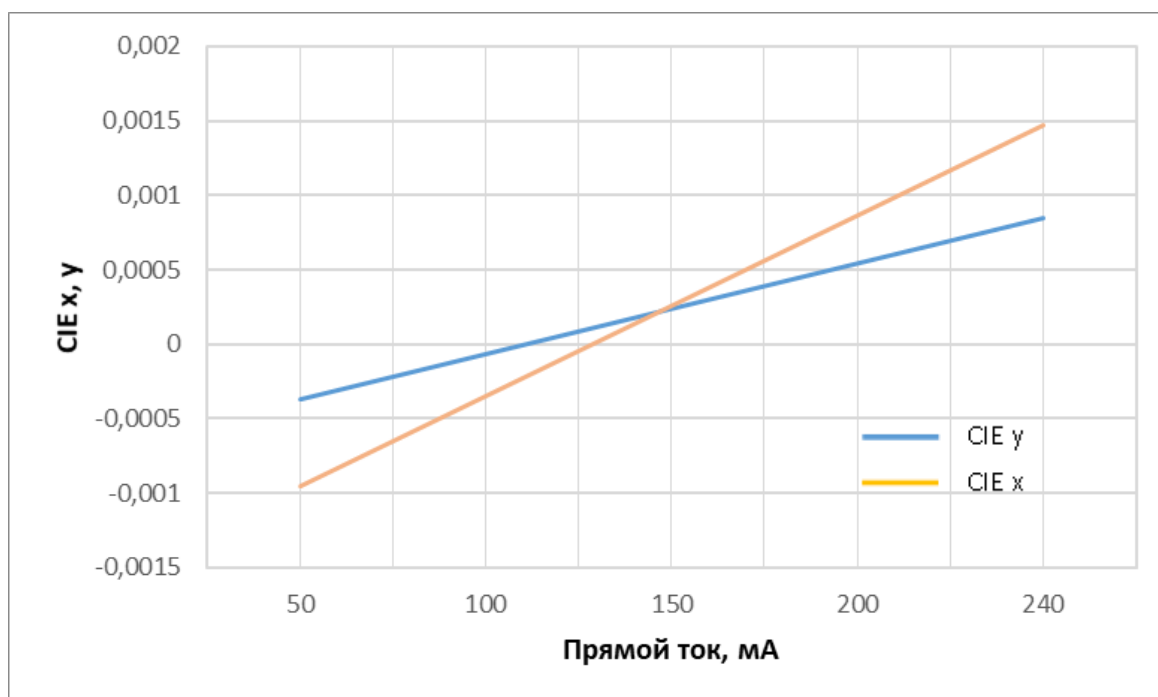
Рисунок 10 – цветковых координат от температуры на контактных площадках ( T_s ) при прямом токе = 150 мА ( I_F )
