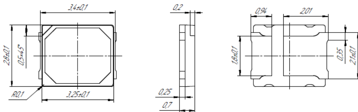
Рисунок 13 – Габаритные размеры Изделия
