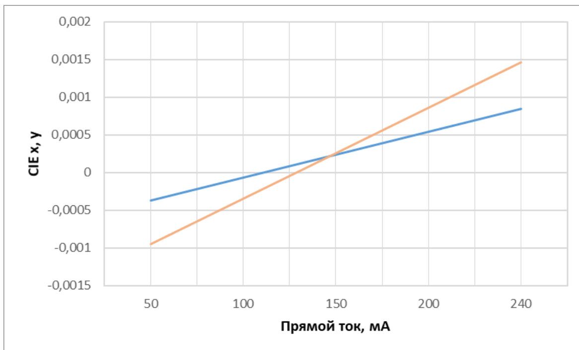
Рисунок 7 – зависимость цветковых координат от прямого тока ( I_F ) при температуре на контактных площадках T_s = 25^\circ\text{C}
