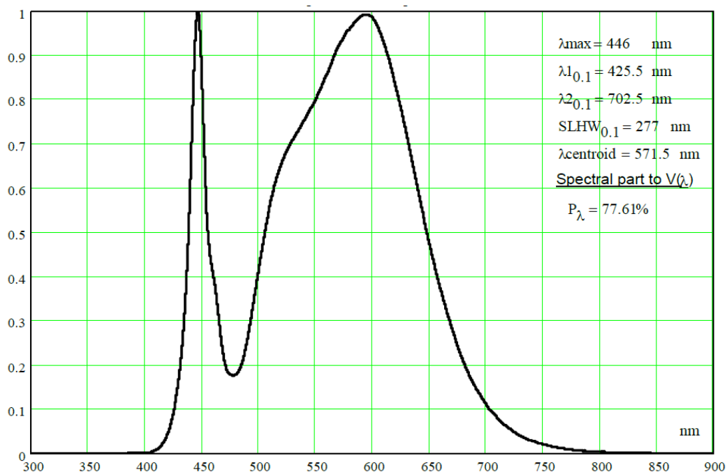
Рисунок 12 – спектр излучения спектр излучения 4000K (при прямом токе 150 мА и температуре на контактных площадках + 25°C)
