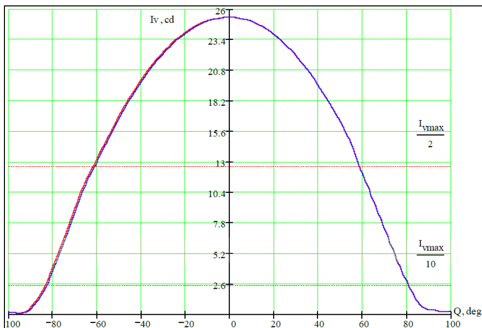
Рисунок 11 – угловое распределение силы света (при прямом токе 150 мА и температуре на контактных площадках + 25°C)
