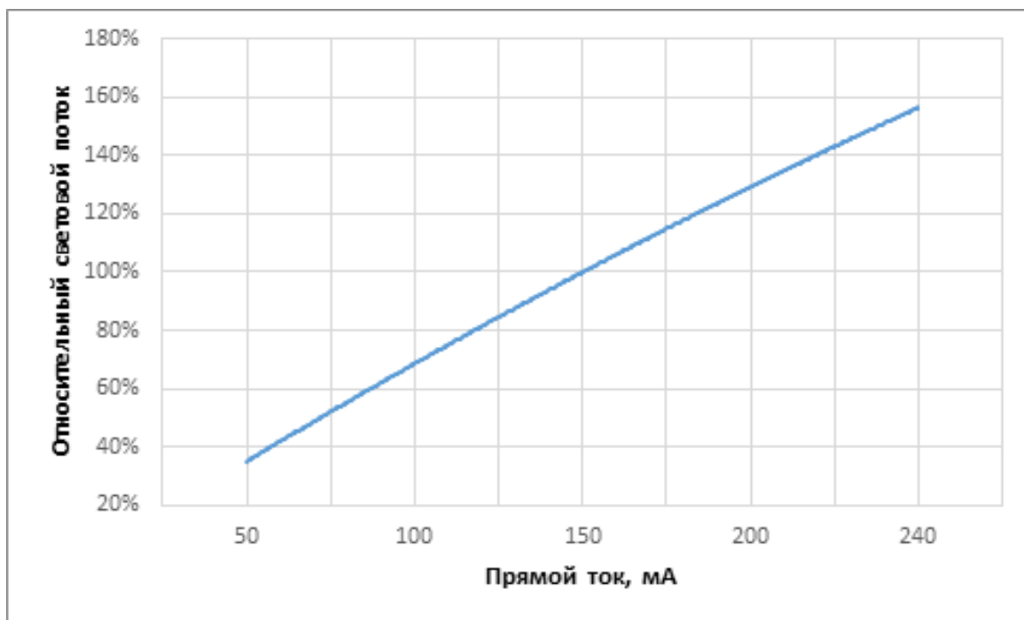
Рисунок 5 – зависимость светового потока от прямого тока ( I_F ) при температуре на контактных площадках T_s = 25\text{ }^{\circ}\text{C}
