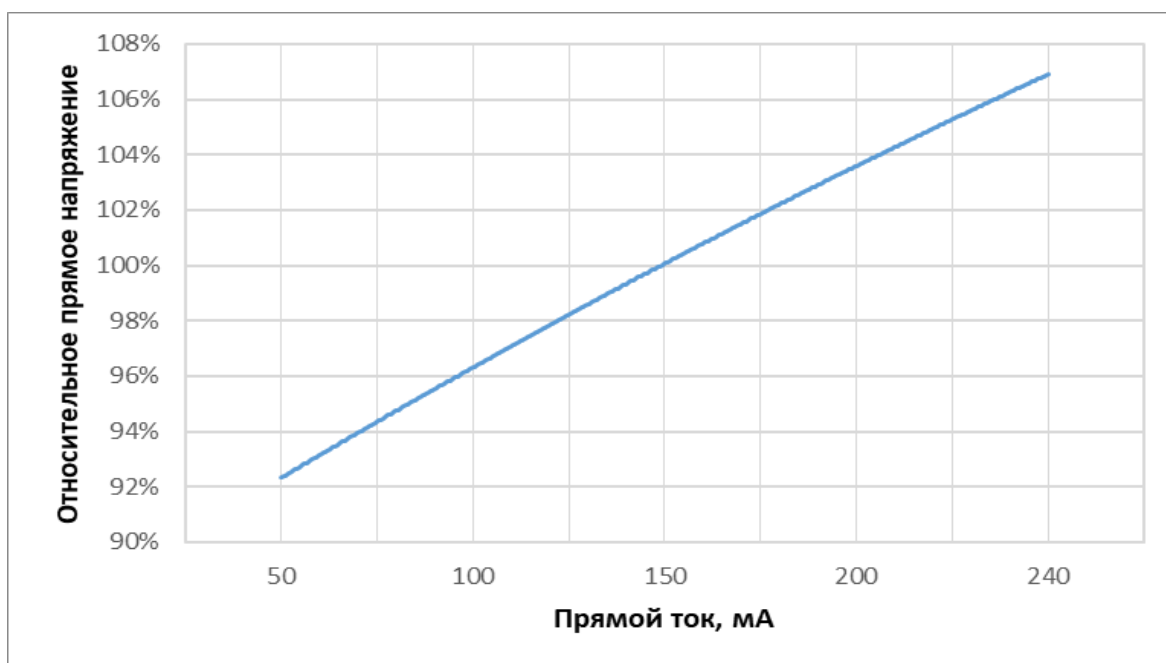
Рисунок 6 – зависимость относительного прямого напряжения от прямого тока ( I_F ) при температуре на контактных площадках T_s = 25\text{ }^{\circ}\text{C}
