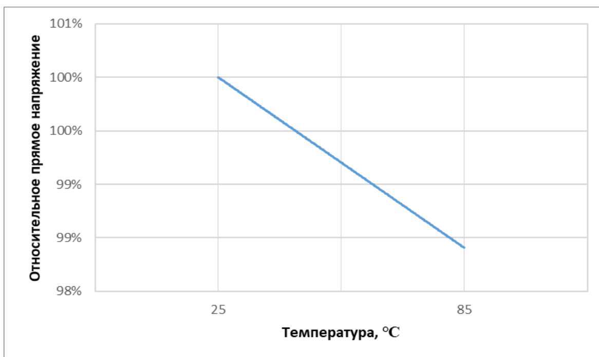
Рисунок 8 – зависимость относительного прямого напряжения от температуры на контактных площадках ( T_s ) при прямом токе = 150 мА ( I_F )
