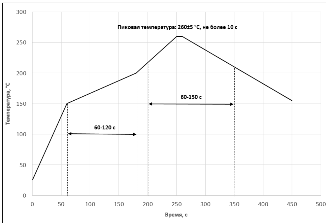
Рисунок 15 – Пример графика температурного профиля пайки
